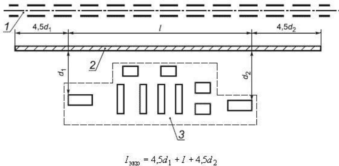
Рисунок 2 - Схема определения требуемой длины акустического экрана
