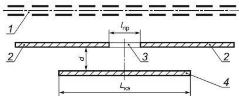
Рисунок 6 - Схема расположения контрэкрана
