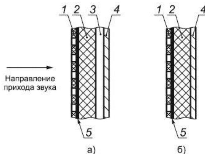
Рисунок 5 - Схема многослойной панели со звукопоглощением с воздушным промежутком и без него
