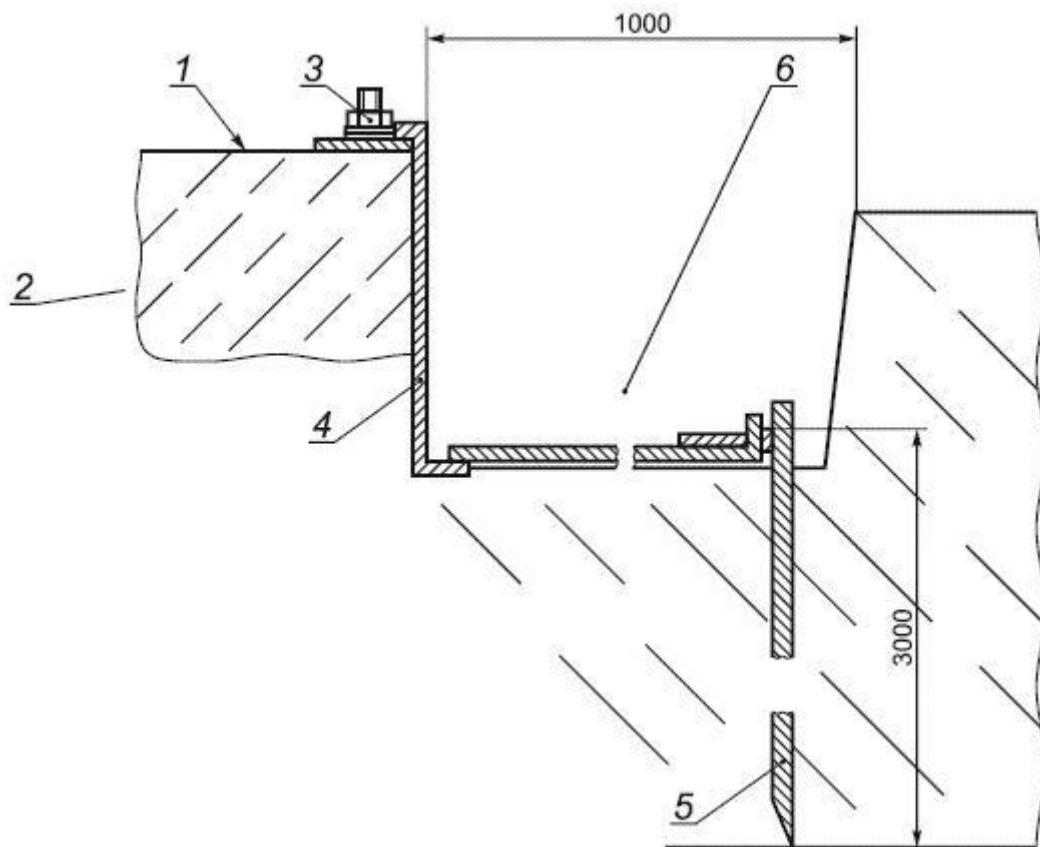
Рисунок 7 - Схема заземления
